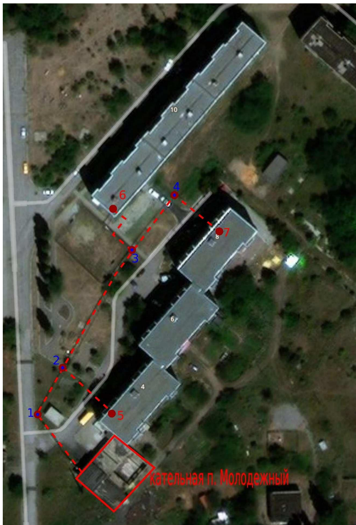
Рис. 1 – Схема тепловых сетей котельной по адресу: п. Молодежный ул. Степная, 4а
