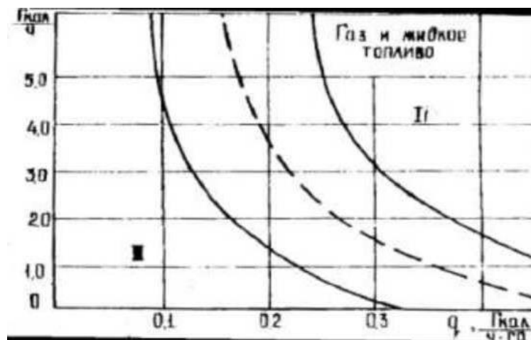
Рис. 3. Ориентировочные значения области устойчивой экономичности централизованного (II) и децентрализованного (I) теплоснабжения.
